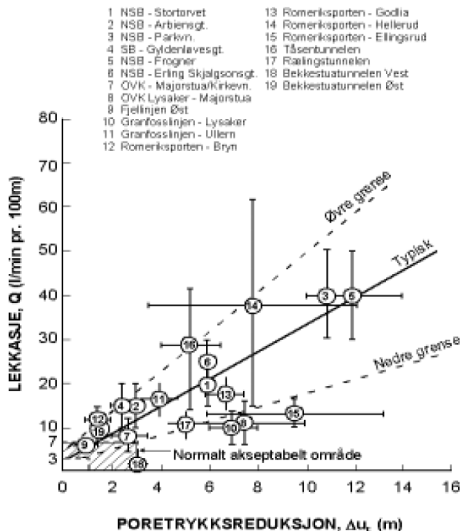
Figur 28: Erfaringskurver for sammenheng mellom innlekkasjerate og poretrykksreduksjon ved berg over tunnel. Hentet fra SVV Publikasjon 103 (Karlsruud, Erikstad and Snilsberg, 2003).
